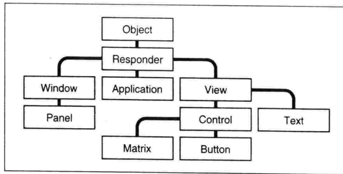
Abb.3: Klassenhierarchie: vorprogrammierte Klassen des »Application-Kit«
