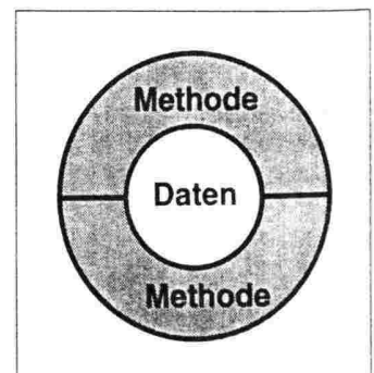
Abb. 1: Ein Objekt: Die Daten sind vollständig von Methoden umschlossen
