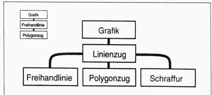
Abb.8: Varianten einer Klassenhierarchie
