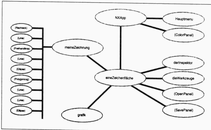
Abb.11: Objekthierarchie des Beispielprogrammes
