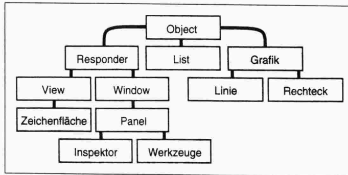
Abb. 5: Klassenhierarchie des Beispielprogrammes
