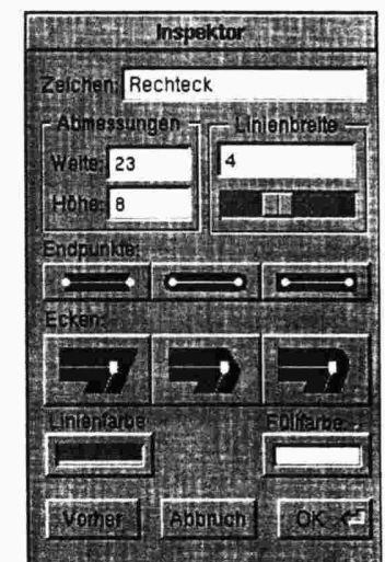
Abb.9: InspektorPanel
