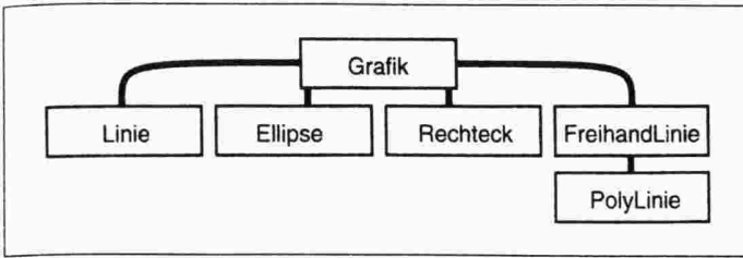
Abb.6: Unterklassen der Superklasse 'Grafik'
